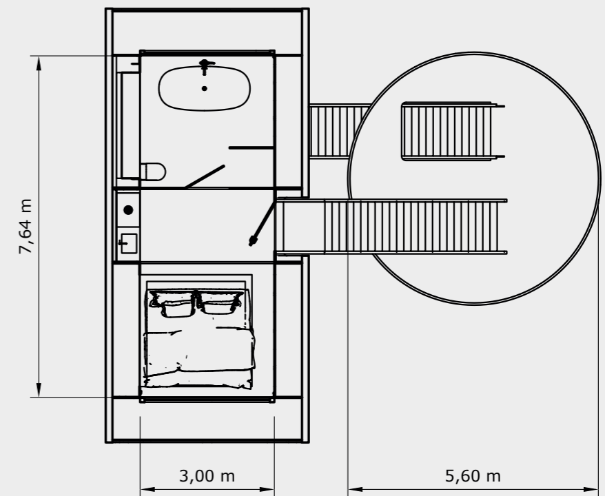
bovenaanzicht
