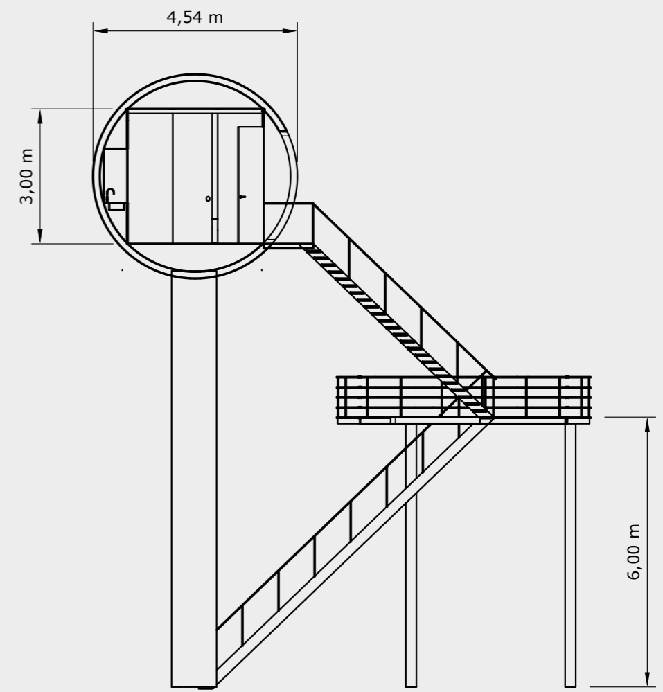
vooraanzicht
